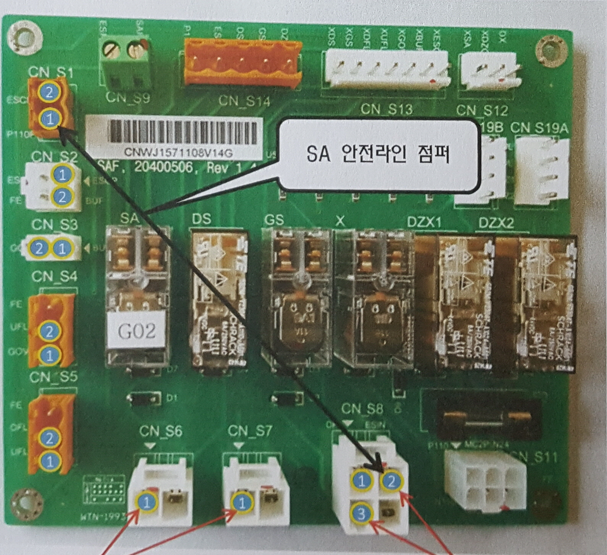
CN_S6-1 [DS] ~CN_S7-1 [DSIN] 승장도어 점퍼 라인 CN_S8-2 [ESIN] ~ CN_S8-3 [GS2] 카도어 점퍼 라인
